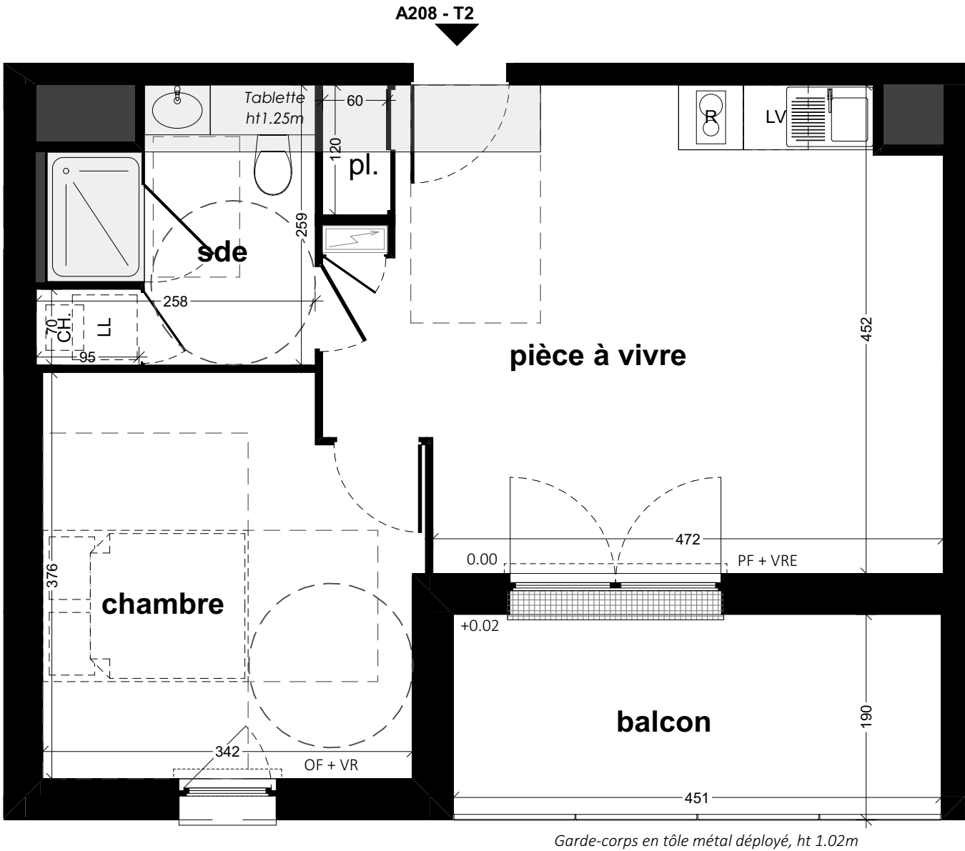
Garde-corps en tôle métal déployé, ht 1.02m
